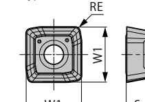
Fig. 4 Centrální destička
