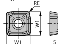
Fig. 3 Centrální destička
