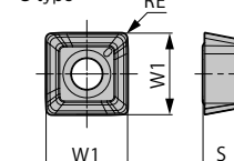
Fig. 4 Centrální destička
