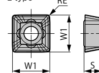
Fig. 3 Centrální destička
