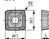
Fig. 3 Inserto Tipo Centrale tipo L
