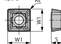
Fig. 1 Inserto Tipo Periferico tipo L
