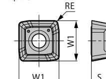
Fig. 4 Inserto Tipo Centrale tipo G
